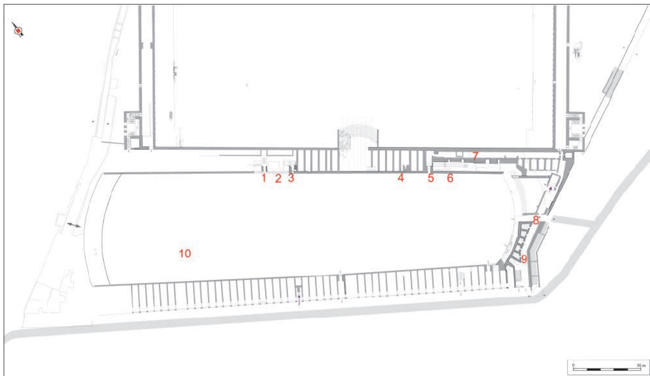
Figura 1. Planta general de les restes conservades del circ en base a la Planimetria Arqueològica de Tàrraco (MACIAS et al. 2007), amb indicació de les intervencions mencionades: 1- Sedassos, 16; 2- plaça dels Sedassos; 3- Sedassos, 24; 4- Trinquet Vell, 12; 5- Trinquet Vell, 16; 6- carrer del Trinquet Vell; 7- carrer de l'Enrajolat; 8- Porta triumphalis ; 9- Voltes de Sant Ermenegild; 10- plaça de la Font.
