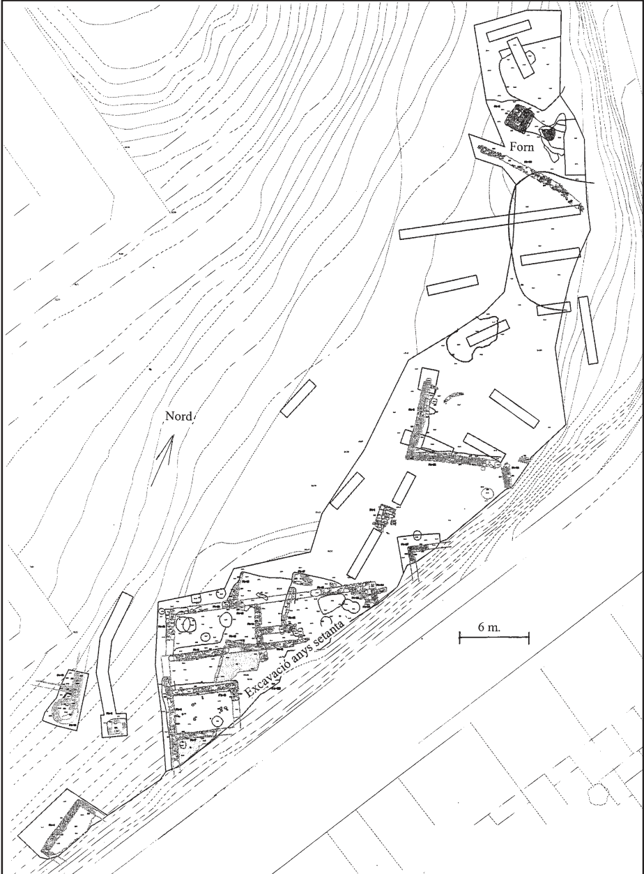
Figura 1.- Planta de les excavacions de la vil·la de Caputxins, que inclou els vestigis trobats l'any 2005 en l'actuació de J. Hernández-Gasch (dibuix: AIA - Museu de Mataró).
