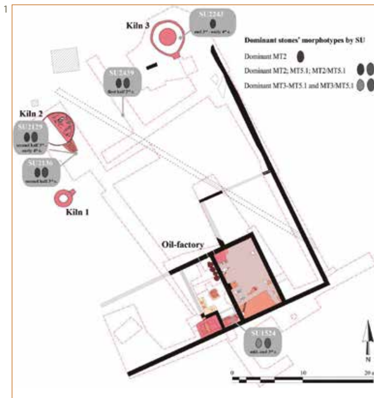
Figura 6. 1-2. Planta de la almazara y alfar de Las Delicias y detalle de uno de sus hornos (Bourgeon et alii , 2018). 3. Reconstrucción de un horno de ánforas oleícolas Dr. 20 realizado por Piero Berni.
