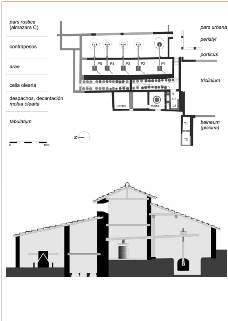
Figura 3. 1. Planta y sección de la almazara de la villa de Milreu. 2. Reconstrucción de la villa (Teichner, 2011-2012).
