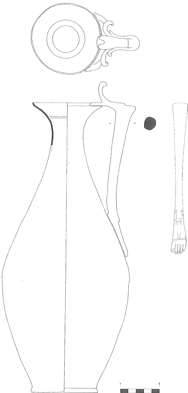
Fig. 5a. Secció i detall del gerro 1.3.
