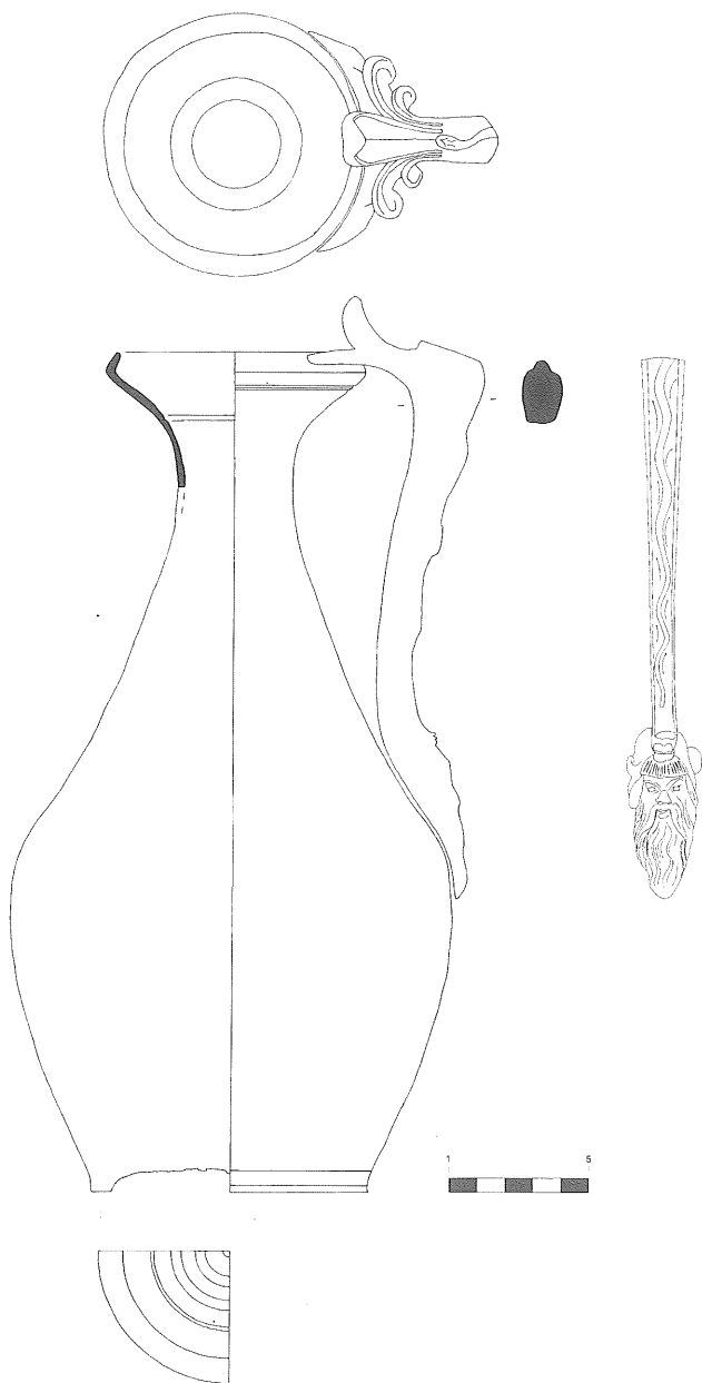
Fig. 6a. Secció i detall del gerro 1.4.
