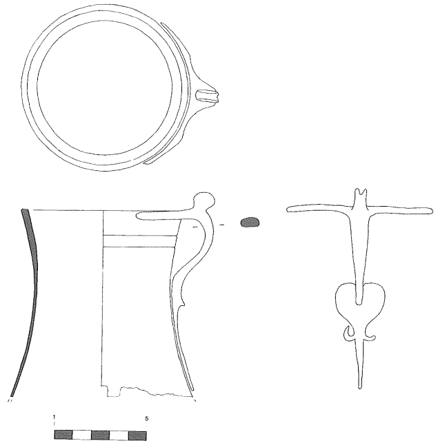
Fig. 21a. Secció i detall del gobelet 5.4.
