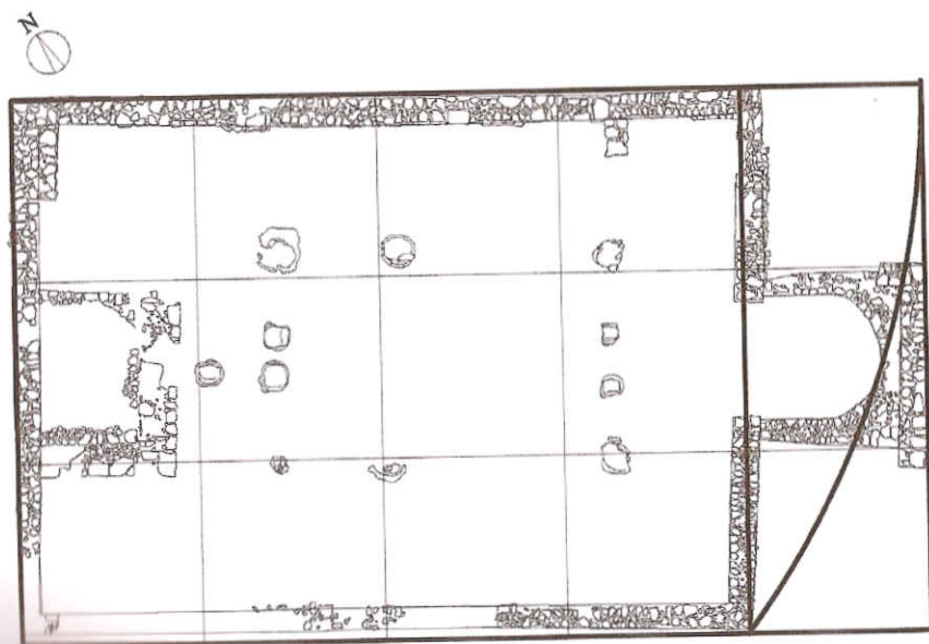
Fig. 3 Disseny arquitectònic de l'església a partir d'un rectangle de raó pitagòrica 3:4:5.
